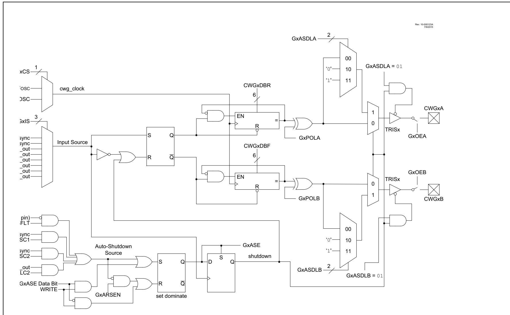
PIC16(L)F1503
